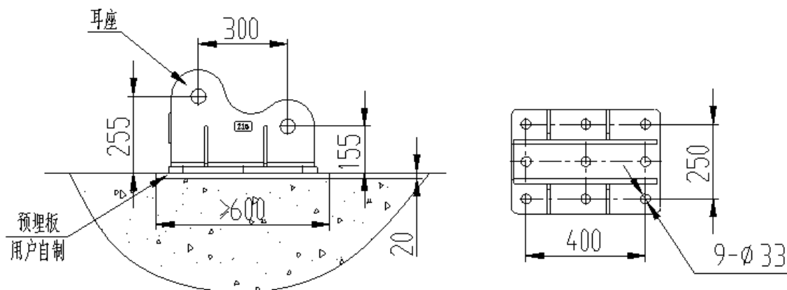
图 4-112 耳座
