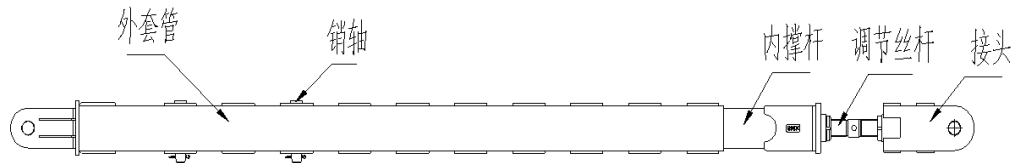
图 4-110 附着撑杆
