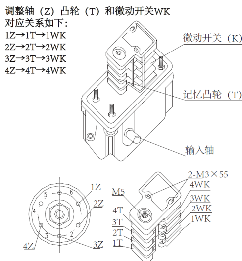
图 4-98 起升限位器图
