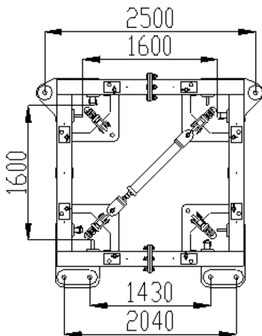
图 4-111 附着框
