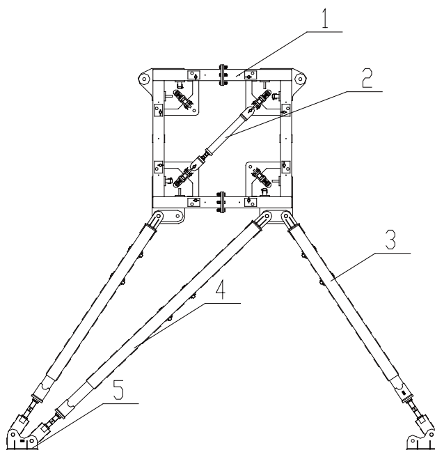
图 4-109 附着架
