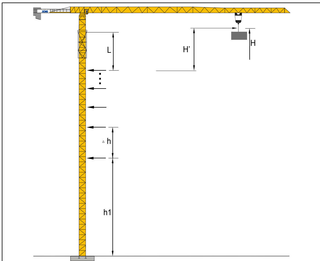
图 4-115 塔机附着示意图
