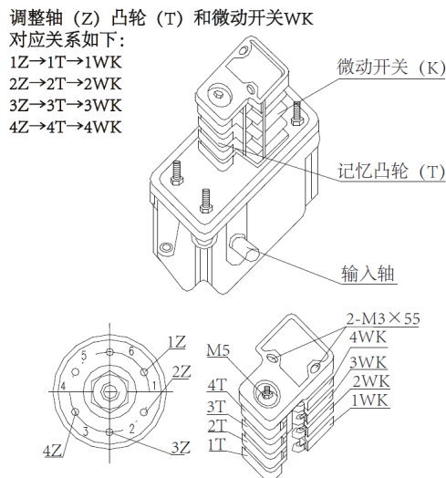
图 4-99 回转限位器图
